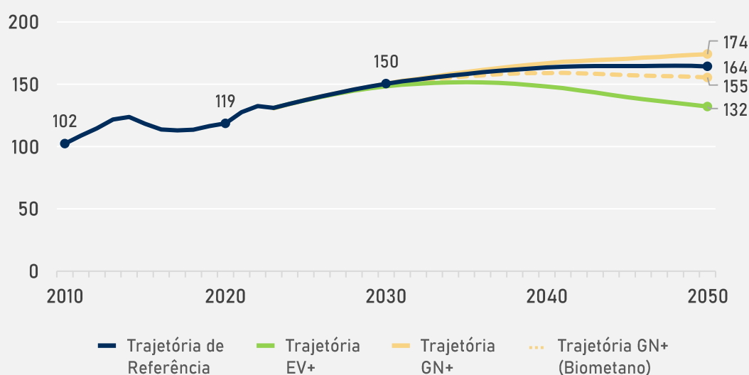
Figura 4-6 Emissões de gases de efeito estufa da frota circulante de veículos pesados no Brasil
