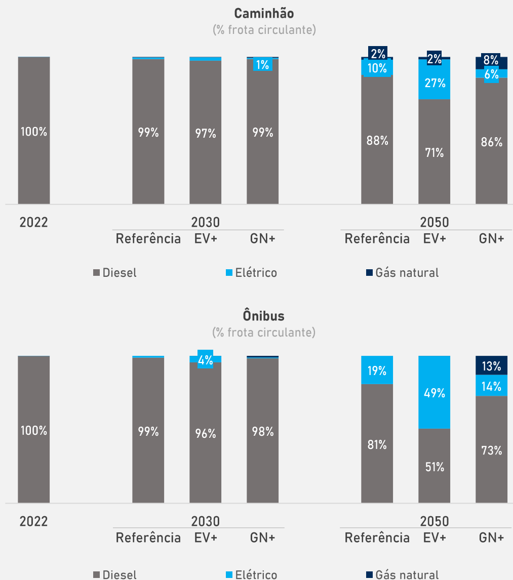
Figura 4-1 Perfil de motorização da frota circulante de caminhões e ônibus no Brasil
