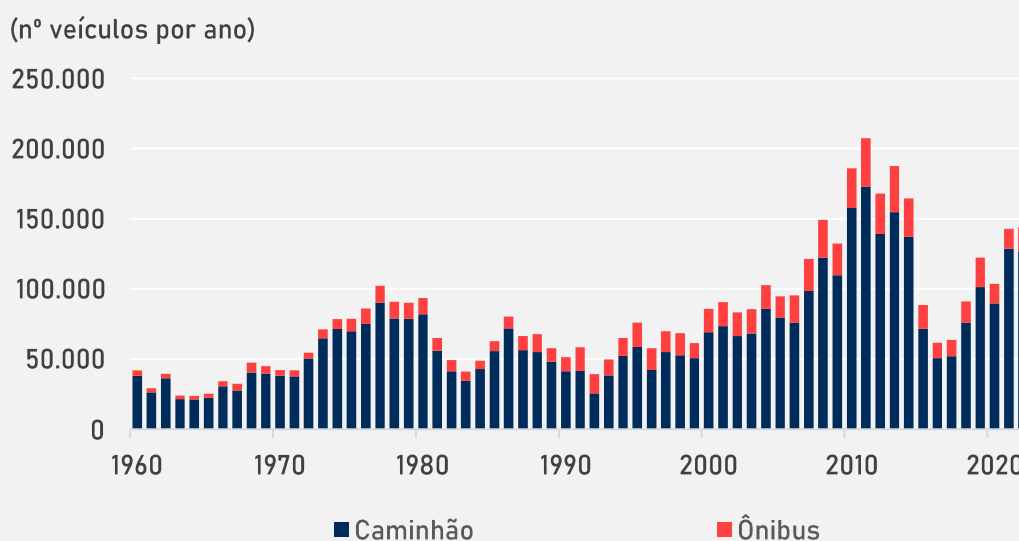
Figura 1-1 Licenciamento anual de caminhões e ônibus novos no Brasil, por tipo de veículo, 1960 - 2022
